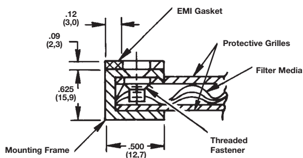
Type 8635
