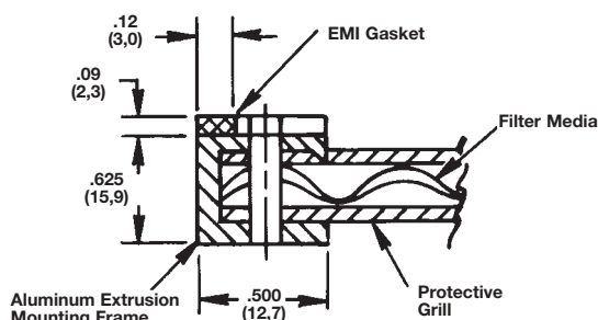
Type 8634
