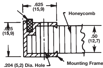
Type 8628
