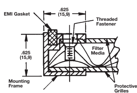
Type 8637
