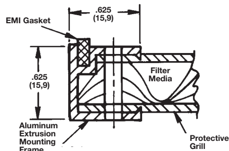
Type 8636
